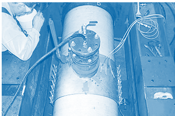
Рисунок 10-12 Испытание давлением скобы и клапанного устройства
