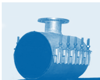
Рисунок 10-11 Рекомендуемые водозаборные скобы для стеклопластиковых труб
