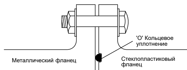
Рисунок 8-4 Фланцевое соединение
