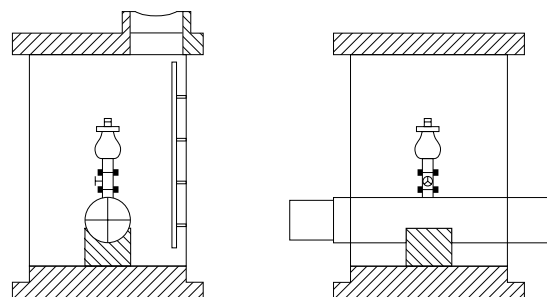
Рисунок 10-2 Клапанные камеры
