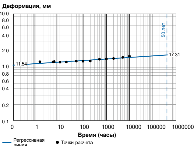
Рисунок 5-8 Долговременная жесткость SN5000 PN 6
