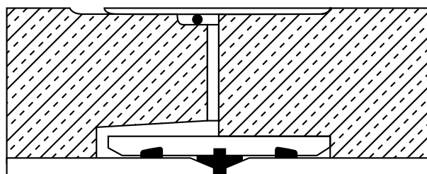
Рисунок 10-10 FLOWTITE система прокола
