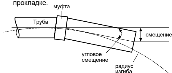
Рисунок 8-3 Максимальное смещение и изгиб трубопровода
