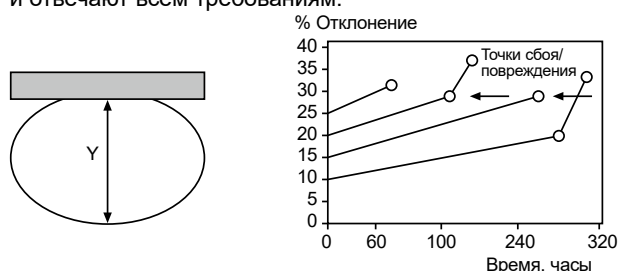
Рисунок 5-5 Влияние долговременного отклонения в воде на эксплуатацию трубы
